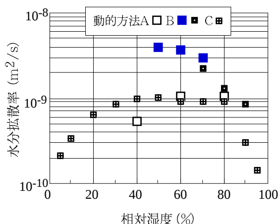
図-2 動的方法によるALCの水分拡散率
