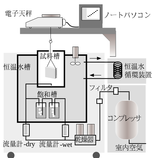
図-1 実験装置の基本構成
