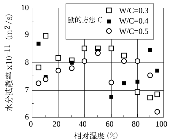
図-4 動的方法CによるHCPの水分拡散率 1)
