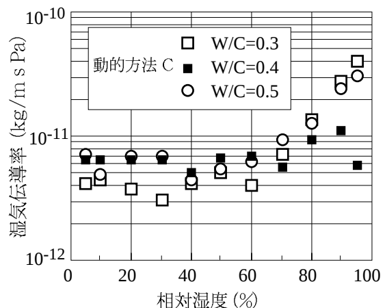
図-5 動的方法CによるHCPの湿気伝導率
